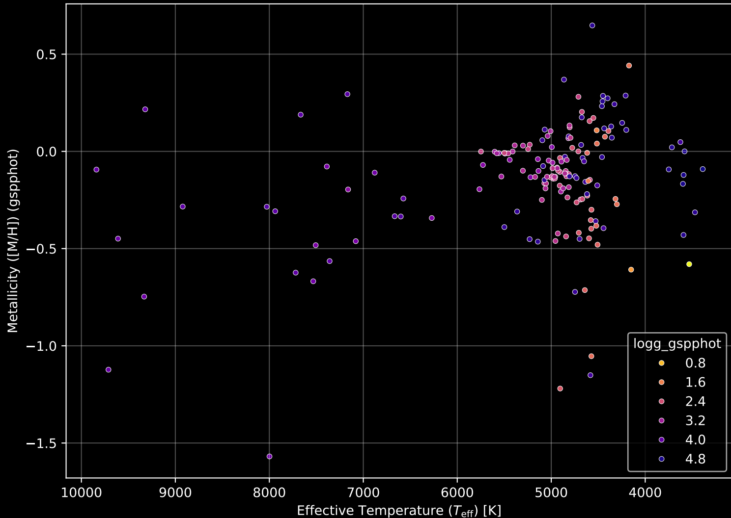
APOGEE DR17 Field: [158+18] Stellar Population Parameters (n= 166)
